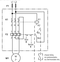
Motores monofásicos Comando à distância
