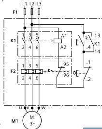
Circuito trifásico para 3TW40 26 e 3TW40 36
