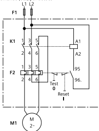
Motores monofásicos Comando local por botões
